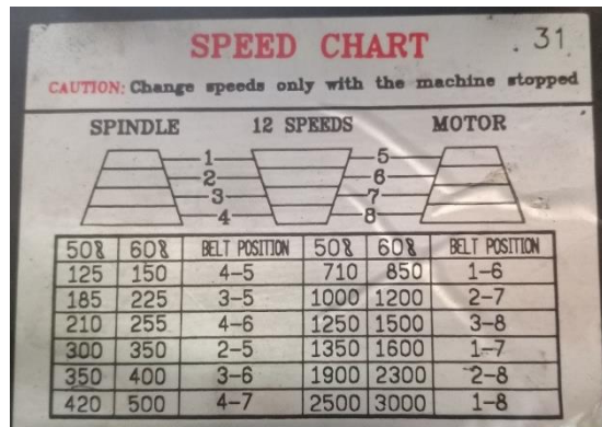
Gambar 1A Variasi kecepatan spindle mesin gurdi
