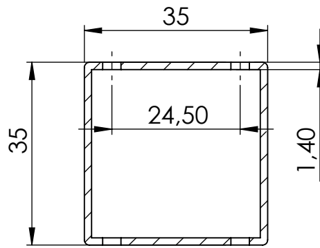
SECTION P-P SCALE 1 : 1
